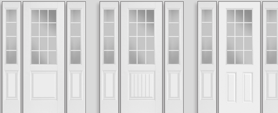
Door: 2248-121-WT58-1 Sidelites: 848-041-WT58-1 Door: 2248-121-WT58-1P Sidelites: 848-041-WT58-1 Door: 2248-121-WT58-2 Sidelites: 848-041-WT58-1
